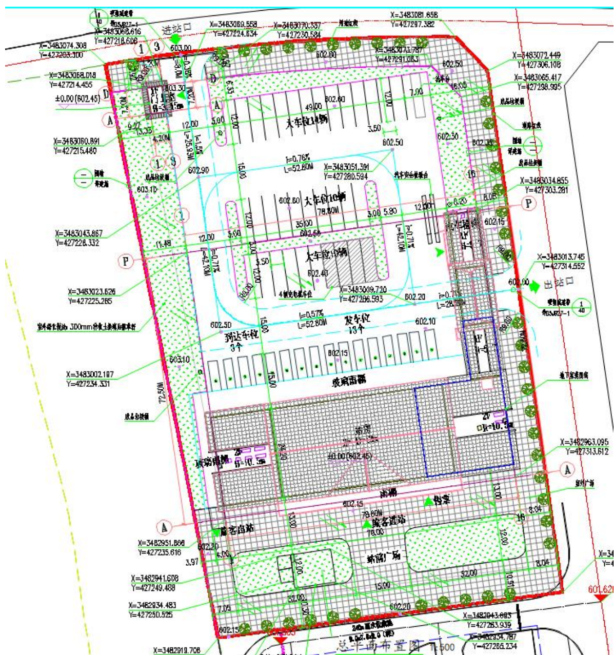
图 2.2-1 项目总平面布置图
